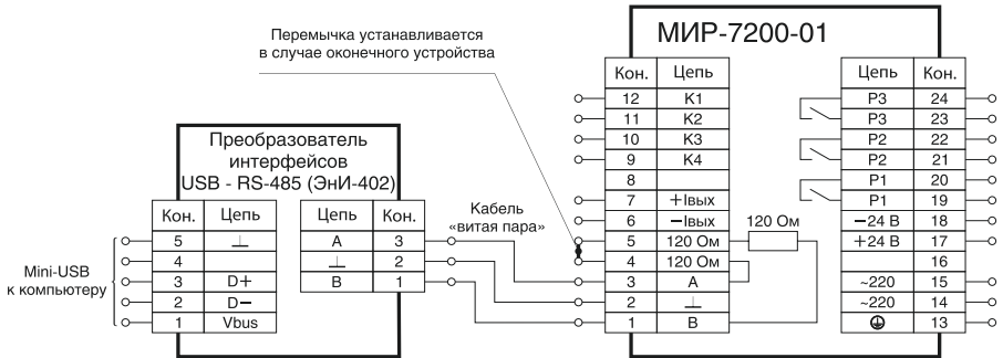
Рисунок Б.11 — Схема подключения регуляторов с интерфейсом RS-485 к компьютеру
