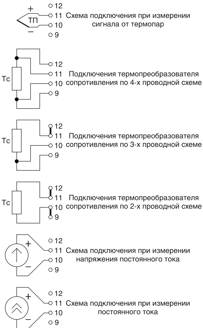
Рисунок Б.4 — Схемы подключений термопар, терморезисторов сопротивления по 4-х, 3-х и 2-х проводным схемам, подключения при измерении напряжения постоянного тока и силы постоянного тока к регулятору исполнения 01
