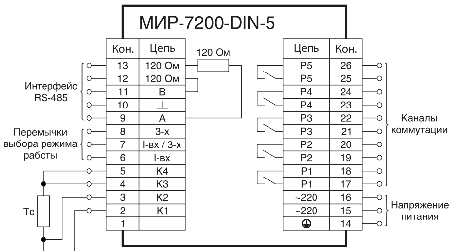
Рисунок Б.8 — Схема подключения к регулятору исполнения DIN с пятью каналами коммутации термпреобразователя сопротивления по четырехпроводной схеме
