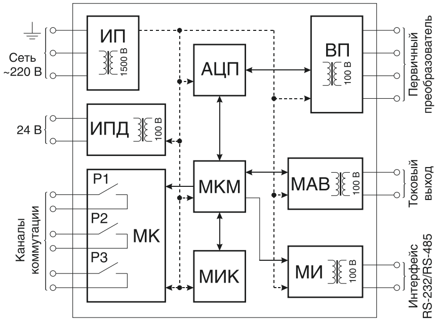
Рисунок 1 — Функциональная схема регуляторов в исполнении DIN и 01
