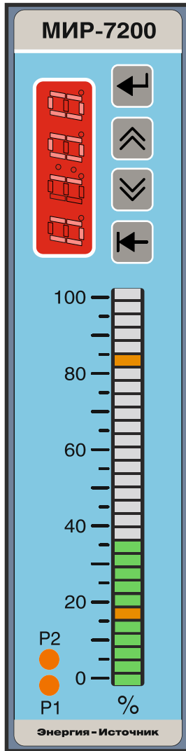
Рисунок А.8 — Внешний вид регулятора исполнения 03 при установке в вертикальной ориентации
