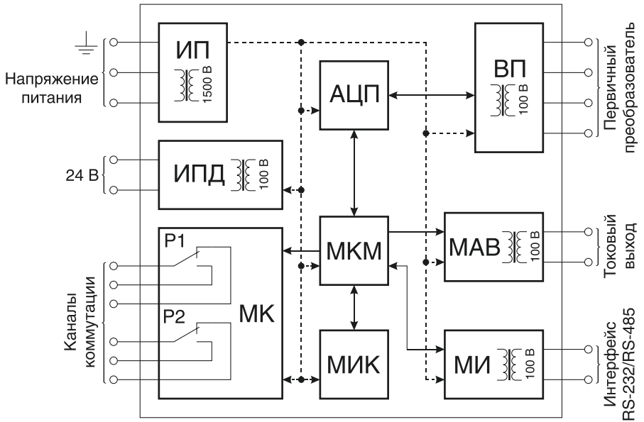
Рисунок 2 — Функциональная схема регулятора в исполнении 02 и 03
